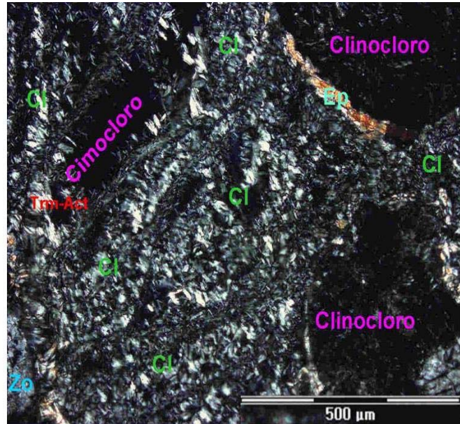
Figura 9. Microfotografía muestra 8. Igual a la foto anterior. (Nicoles cruzados). 10x.
